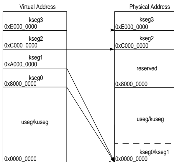
Figure 6 FMT Memory Map (ERL=1) in the 4KEp Core
