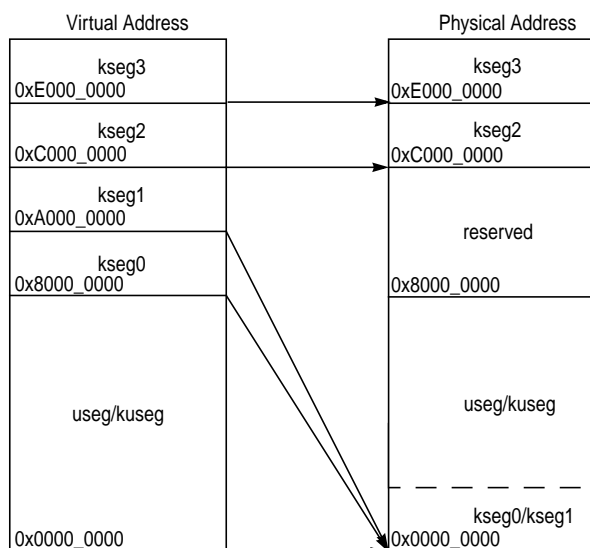
Figure 6 FMT Memory Map (ERL=1) in the 4KEM Core
